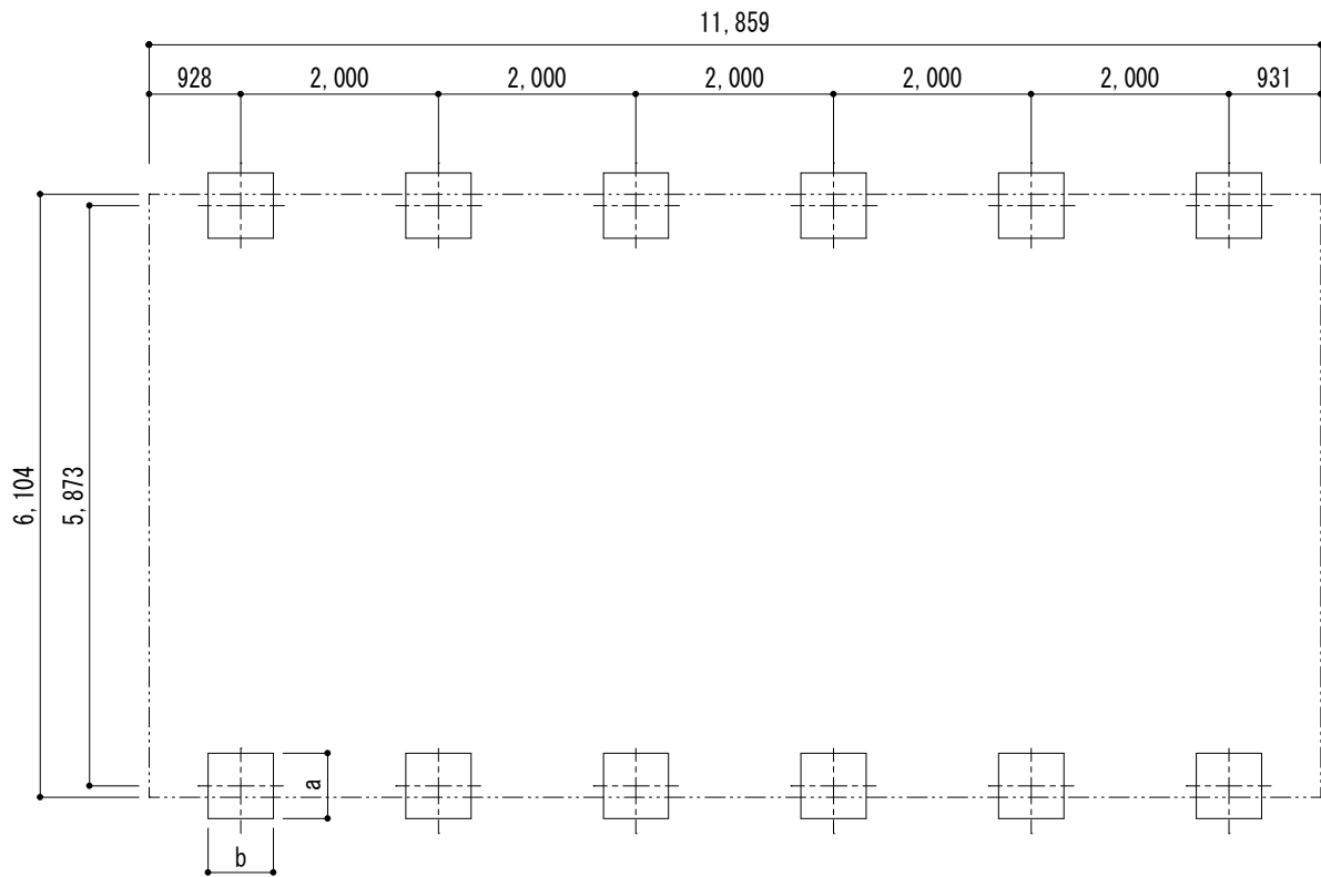
■基礎配置図
